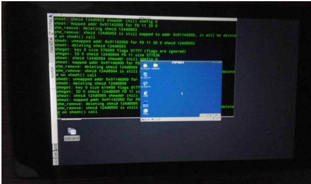
Windows9x、2000
