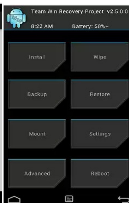
TWRP
